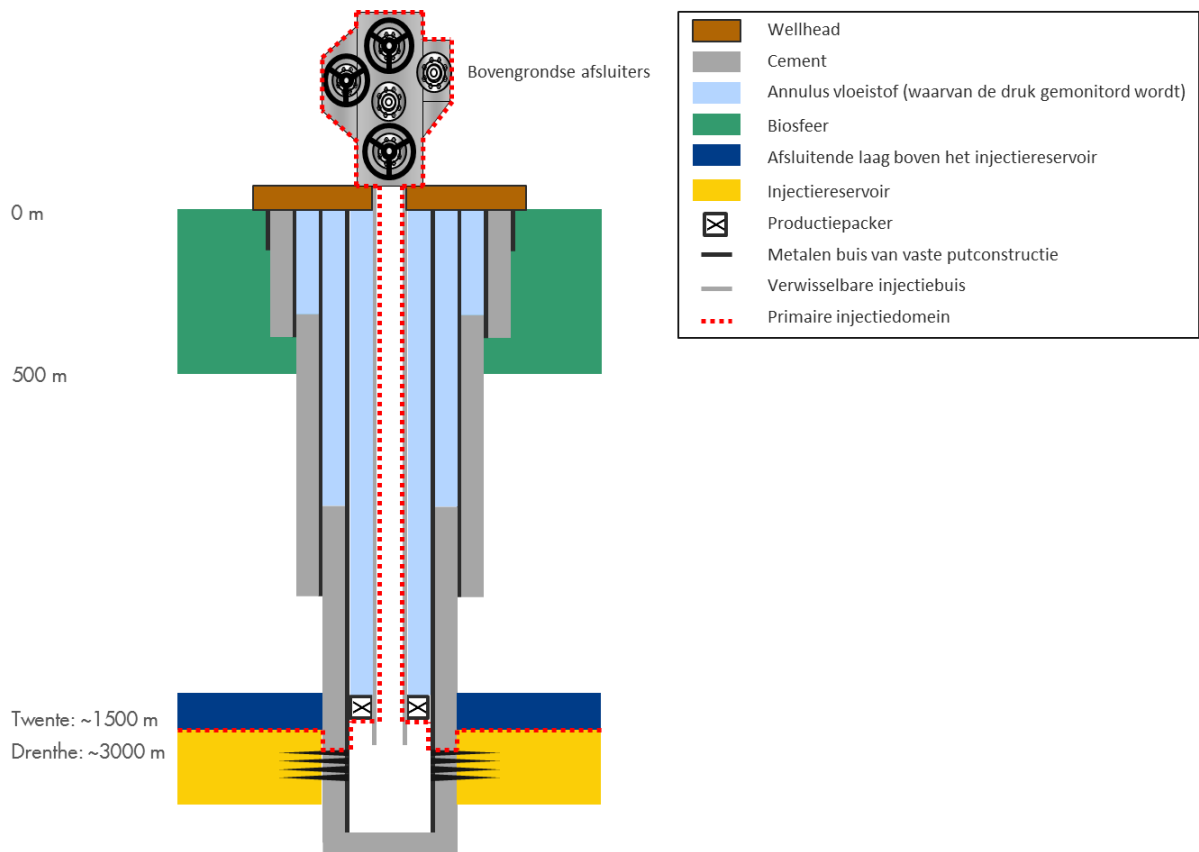
Figuur 5: Schematische weergave van een typische putconstructie
