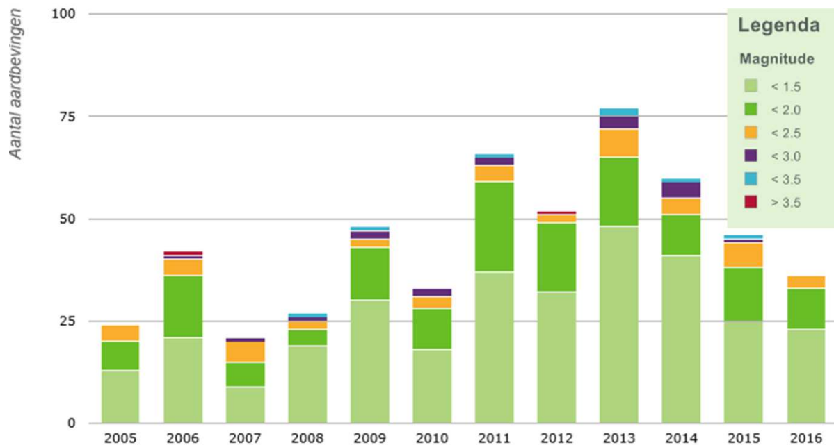
Figuur 2 ontwikkeling seismiciteit Groningen veld 2005 – 2016 exclusief magnitudes kleiner dan 1.0; opmerkelijk is de reductie van het aantal bevingen sedert de productie ingrepen vanaf 2014
