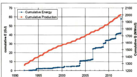
Figuur 2. Sterke toename van de vrijgekomen hoeveelheid seismische energie in de tijd, voornamelijk door aardbevingen met een grotere sterkte dan 3 (Richter) vanaf 2003.
