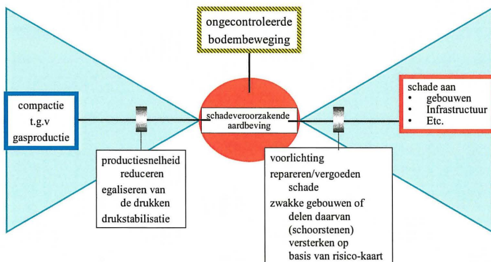
Figuur 3. Vlinderstrik diagram. In de knoop van de strik staat de ongewenste gebeurtenis vermeld: een schadeveroorzakende aardbeving.
