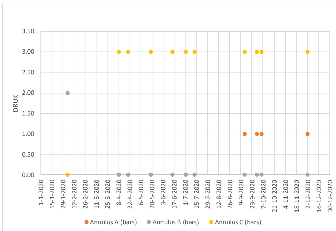
Figuur 1: SLD-01 annulus drukken in 2020.
