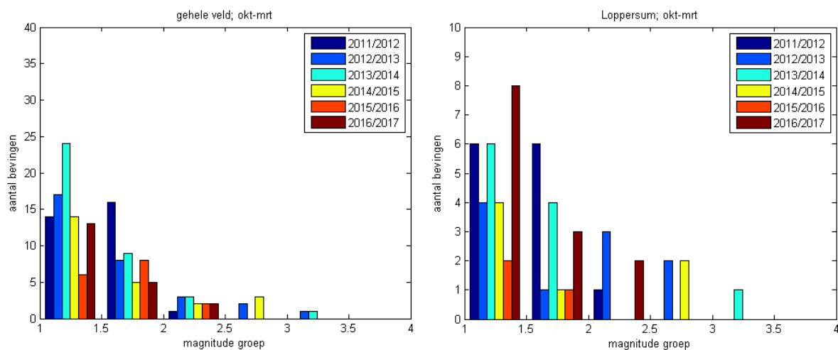
Figuur 2: Aantal aardbevingen \geq 1,0 in de winter periode van het gasjaar (oktober t/m maart) voor links het gehele Groningen gasveld en rechts de regio rond Loppersum.
