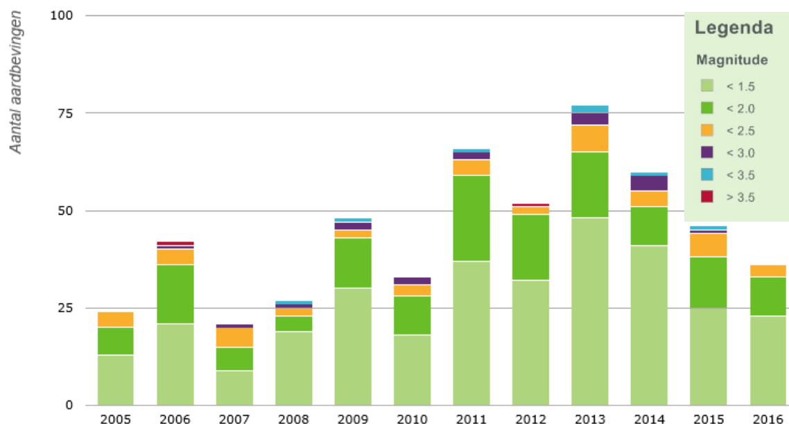
Figuur 1: Aantal aardbevingen \geq 1.0 in het Groningenveld van 2005 tot 2016
