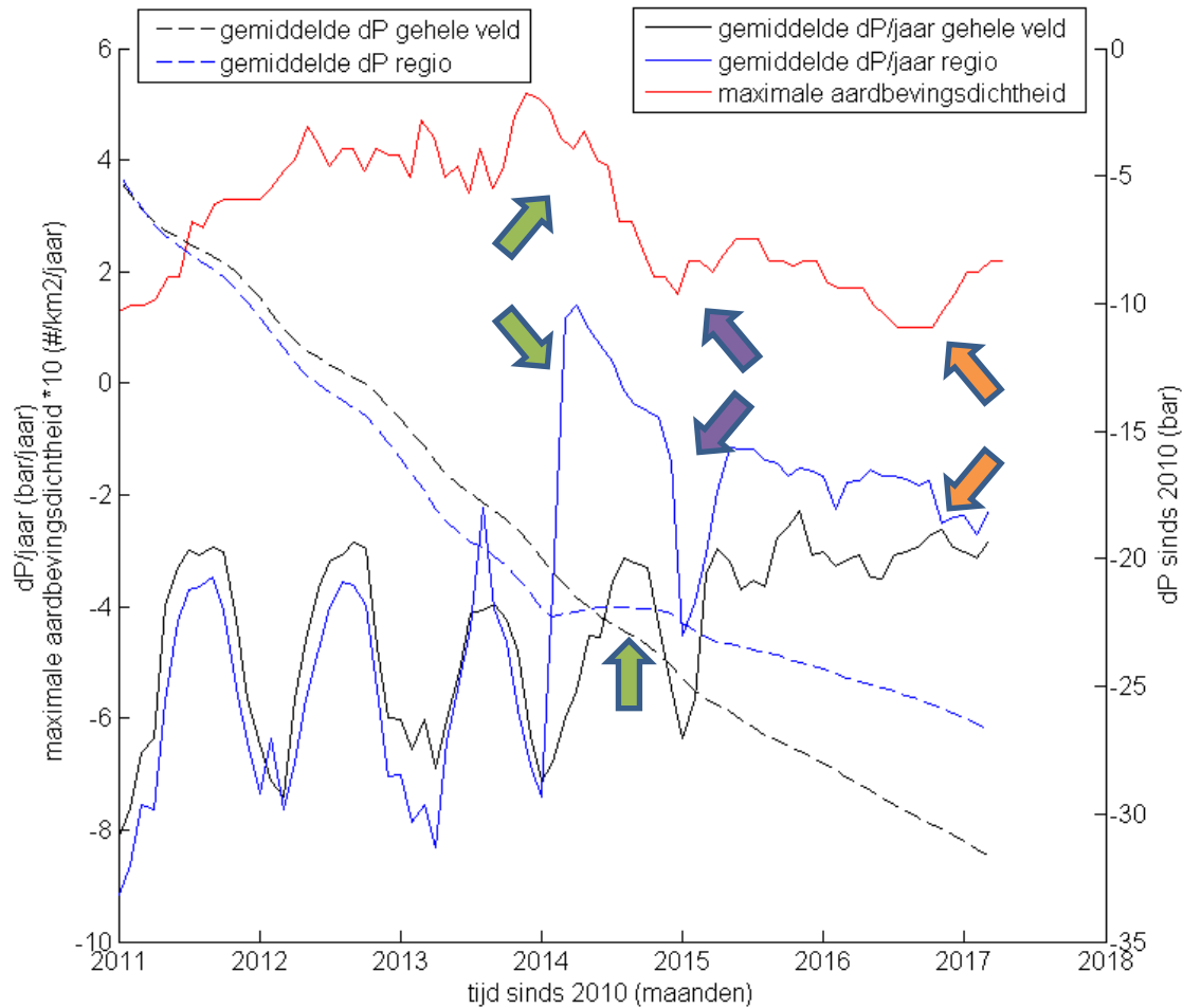
Figuur 8. De ontwikkeling van de drukdaling, de snelheid van drukdaling (verandering in drukdaling ten opzichte van de voorgaande maand) (blauwe lijnen) en de maximale aardbevingsdichtheid (rode lijn) in de regio Wirdum. Ter referentie is ook de ontwikkeling van de drukdaling en snelheid van drukdaling gemiddeld over het hele Groningen gasveld weergegeven (zwarte lijnen).
