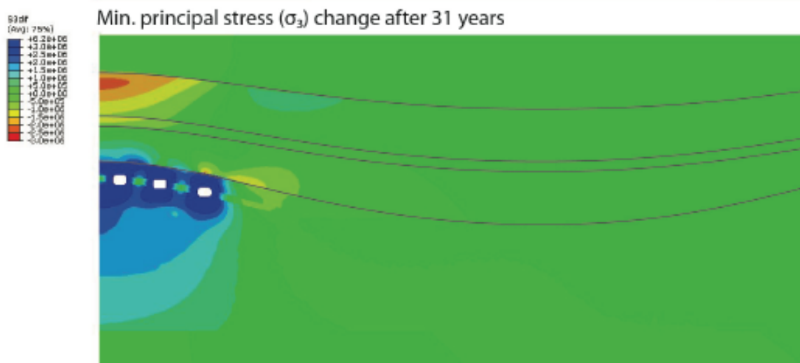
Figuur 7: Verandering in de min principal stress in Pa voor een plain strain benadering door . De spanningsveranderingen in het zout bedragen tot 60 bar ( 6 \cdot 10^6 Pa). Het plusteken wordt veroorzaakt doordat in Abaqus drukspanningen negatief zijn en minder negatief worden (dus lager in absolute waarde)
