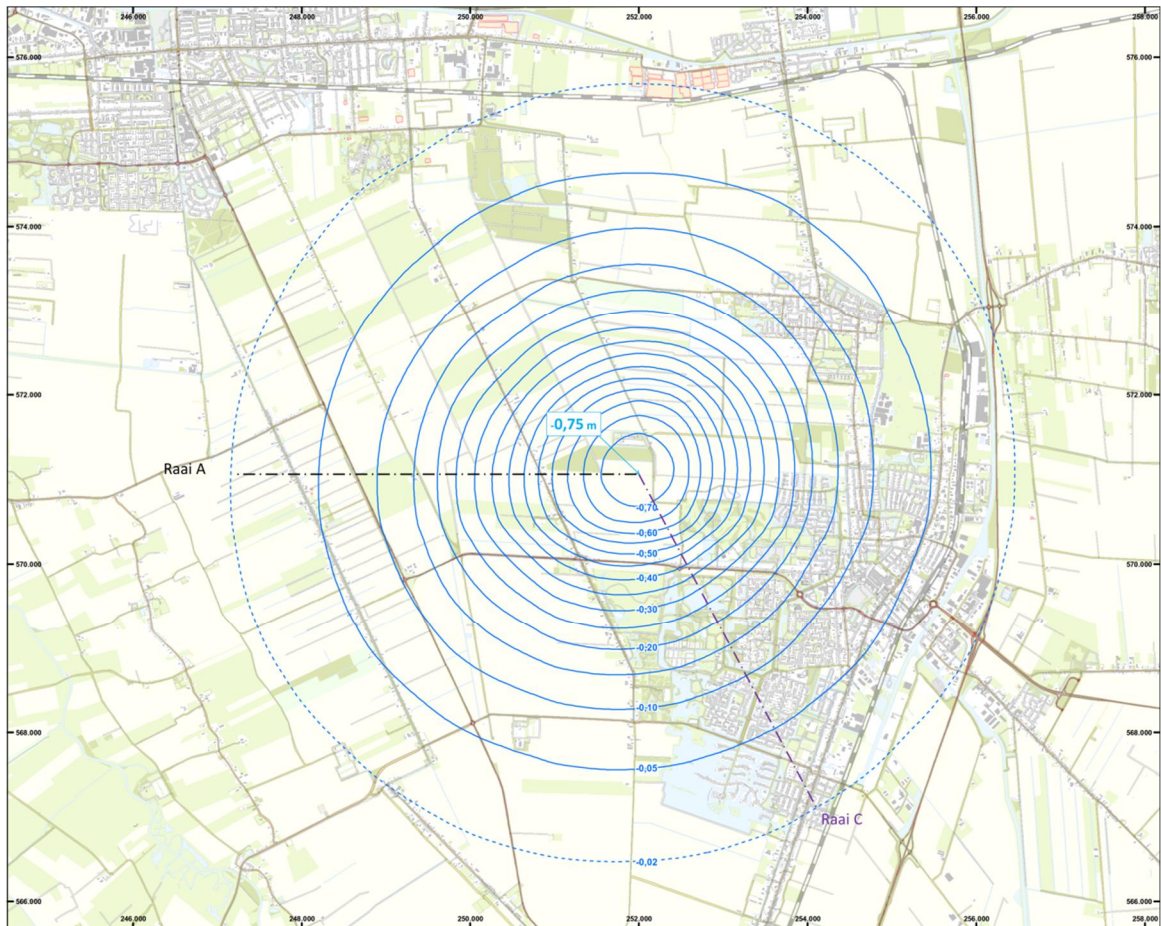
Figuur 4.1 Bodemdalingsgebied met een maximale bodemdaling van 0,75 m (vanaf 1972) [15] met daarin liggend raai A en C
