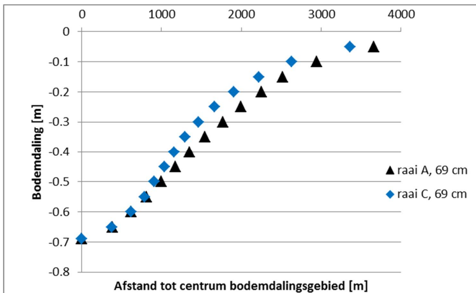
Figuur 3.3 Bodemdaling bij maximale bodemdaling van 0,69 m (vanaf 1972) [5] ter plaatse van raai A en C
