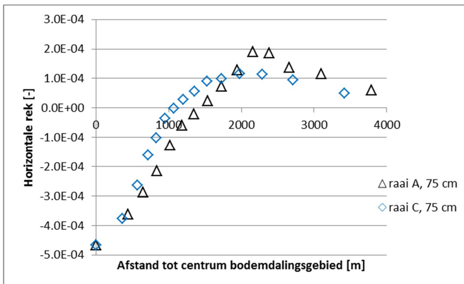
Figuur 4.4 Maximale horizontale rek ter plaatse van raai A en C van het maaiveld bij een bodemdalingsgebied met een maximale bodemdaling van 0,75 m [15]
