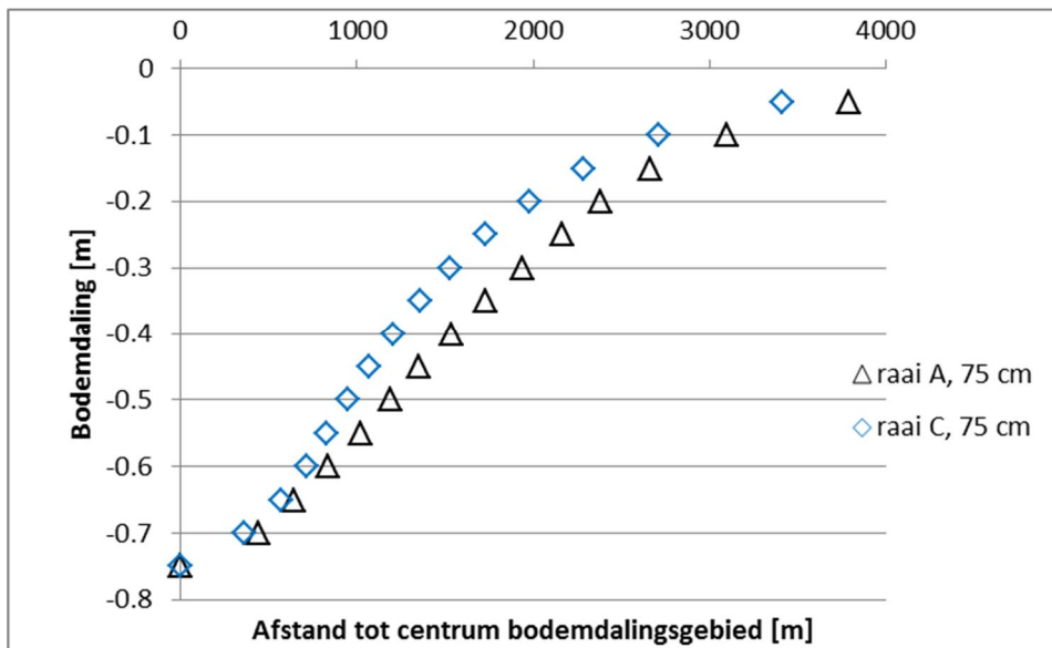
Figuur 4.2 Bodemdaling bij maximale bodemdaling van 0,75 m (vanaf 1972) [15] ter plaatse van raai A en C
