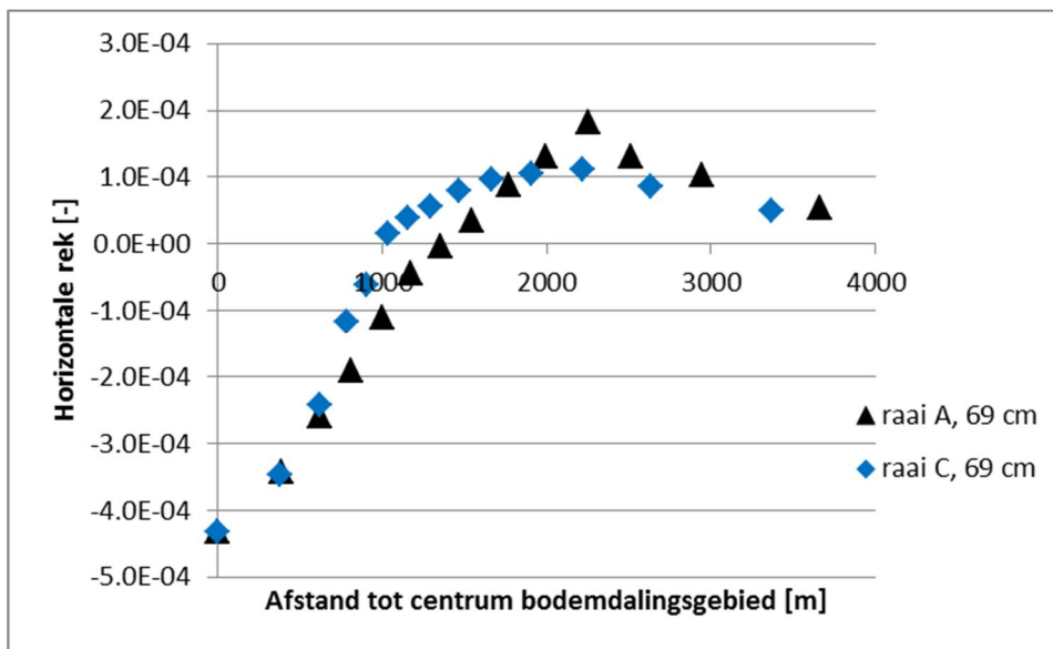
Figuur 3.5 Maximale horizontale rek ter plaatse van raai A en C van het maaiveld bij een bodemdalingsgebied met een maximale bodemdaling van 0,69 m [5]
