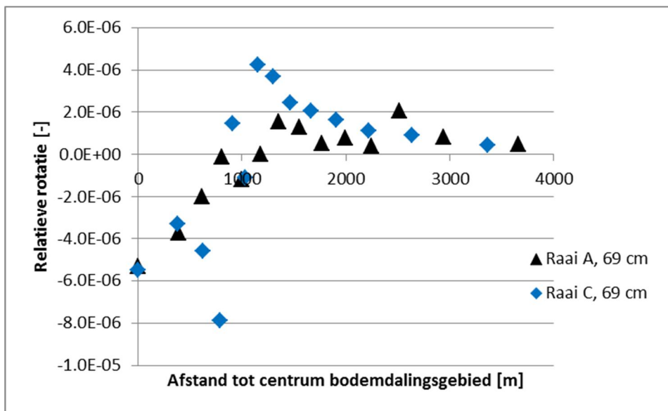
Figuur 3.4 Relatieve rotatie ter plaatse van raai A en C van maaiveld voor gebouw lengte van 20 m in het bodemdalingsgebied met maximale bodemdaling van 0,69 m [5]
