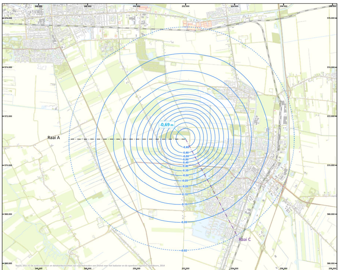
Figuur 3.2 Bodemdalingsgebied met een maximale bodemdaling van 0,69 m (vanaf 1972) [5] met daarin ligging raai A en C
