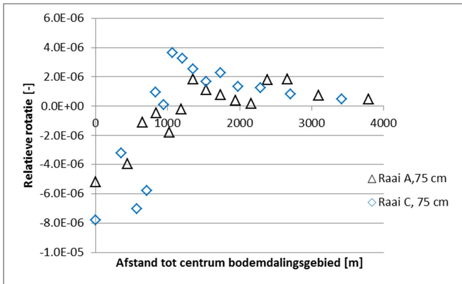
Figuur 4.3 Relatieve rotatie ter plaatse van raai A en C van maaiveld voor gebouw lengte van 20 m in het bodemdalingsgebied met maximale bodemdaling van 0,75 m [15]
