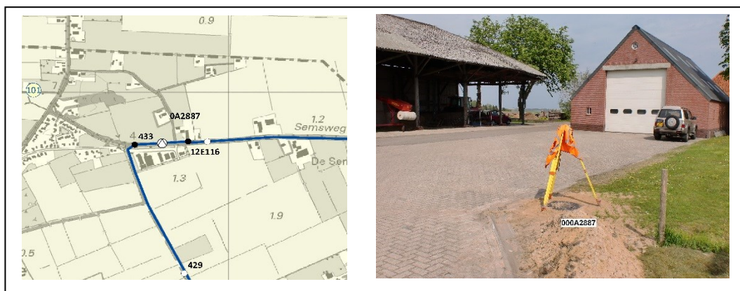
Figuur 1 NAP-peilmerk 000A2887 (ondergronds peilmerk) gesitueerd westelijke rand van het meetnet
