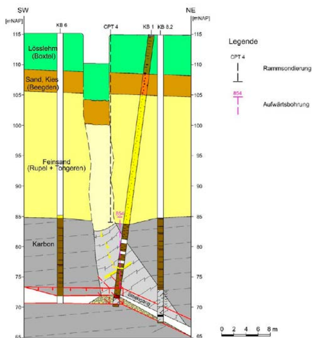
Figuur 37 Sectie met verkenningboringen, sinkhole (midden) en schuine steenhelling waar los materiaal kon wegstromen (bron ingenieursbureau IHS-gemeente Kerkrade).
