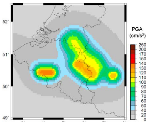
Figuur 53 Inschatting van de seismische hazard in het zuiden van Nederland (De Vos, 2010). Gegeven is de grondversnelling met een overschrijdingskans van 10% in 50 jaar. Dit soort kaarten gaat gepaard met grote onzekerheden en moeten daarom met zorg gebruikt worden.
