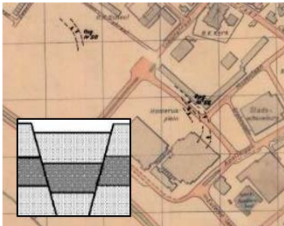
Figuur 28 Sectie met sinkhole aan het oppervlak bij F1. Zie rechts boven de drempels. De schuine laag V onder in het Carboon, waar los materiaal kon wegstromen in de ondiepe industriële winning. Zie ook het mijnwaterniveau dicht bij de overgang van Carboon naar het bovenliggende dekterrein, Maastricht-formatie (bron ingenieursbureau IHS).
