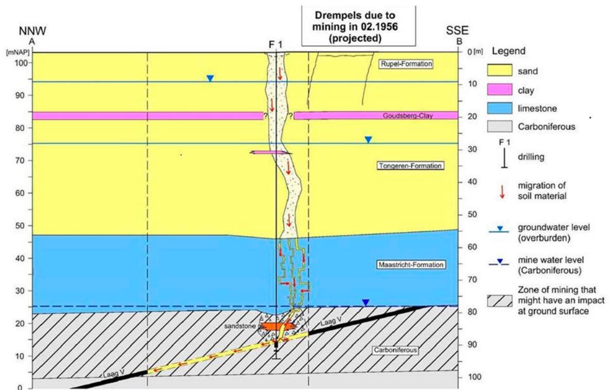
Figuur 28 Sectie met sinkhole aan het oppervlak bij F1. Zie rechts boven de drempels. De schuine laag V onder in het Carboon, waar los materiaal kon wegstromen in de ondiepe industriële winning. Zie ook het mijnwaterniveau dicht bij de overgang van Carboon naar het bovenliggende dekterrein, Maastricht-formatie (bron ingenieursbureau IHS).
