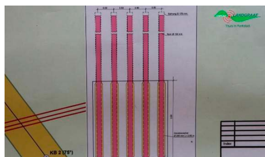
Figuur 39 Patroon van boringen om een dam aan te brengen in de schuine galerij (steenhelling).
