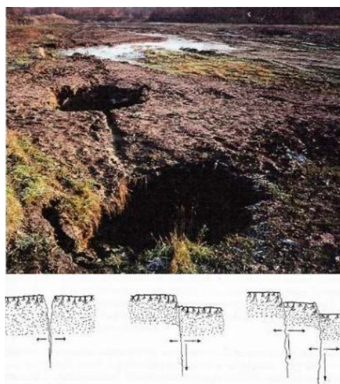
Figuur 12 Een extreem voorbeeld van een scheur door horizontale rek in de fase van intensieve steenkoolwinning, destijds in Duitsland (met kleine sinkholes langs de scheur).
