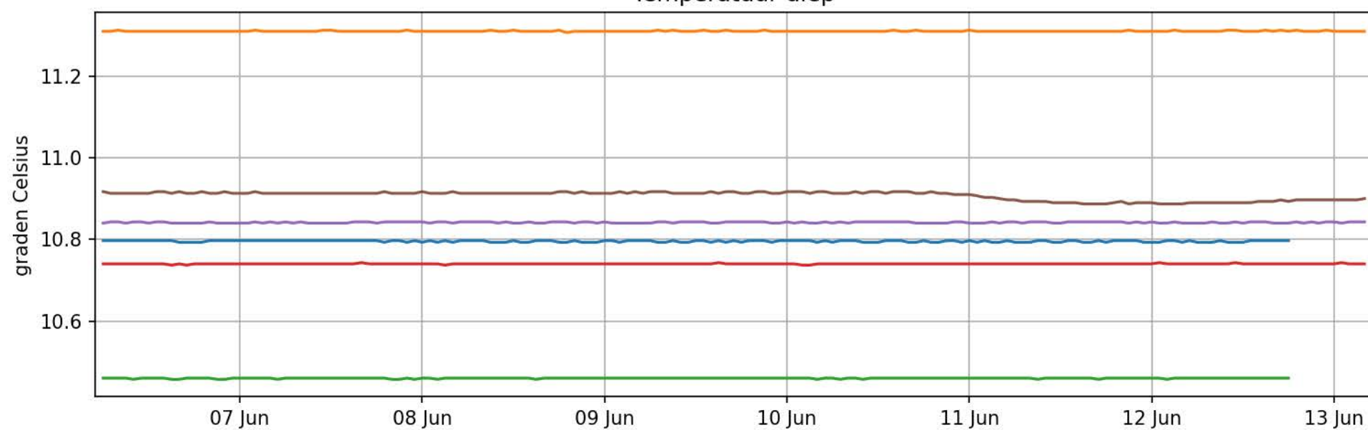
Temperatuur diep
