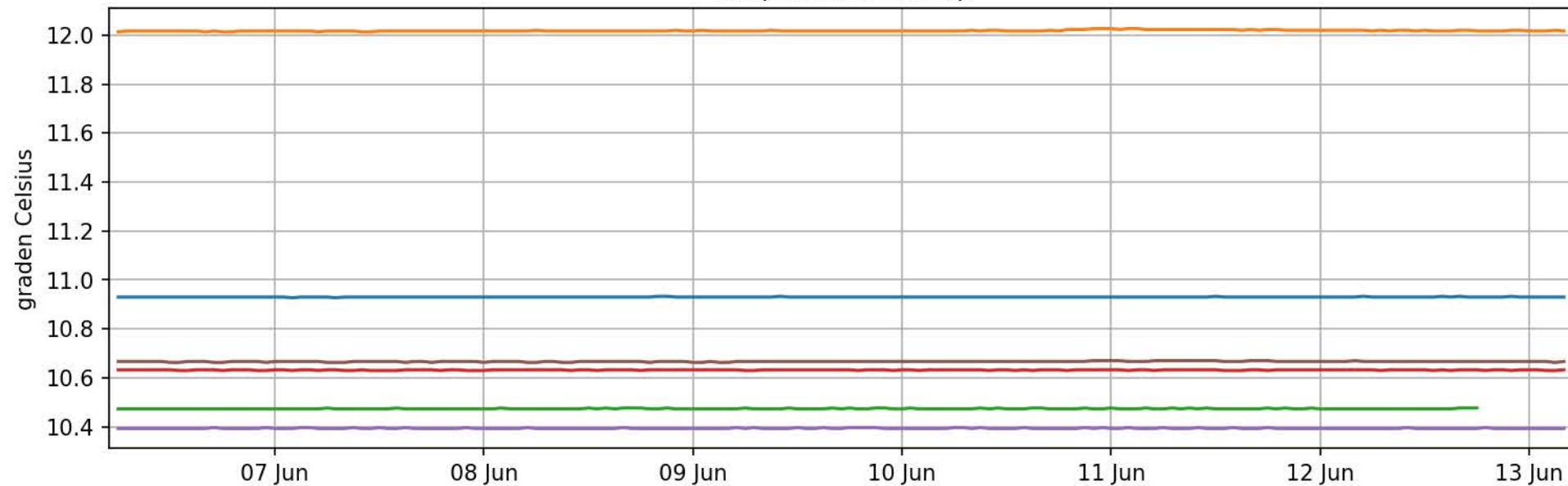
Temperatuur diep
